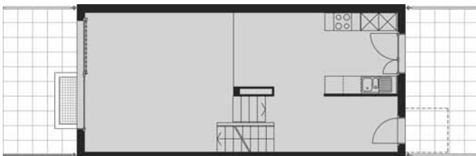
Plan du rez-de-chaussée
