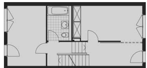
Plan d'étage
