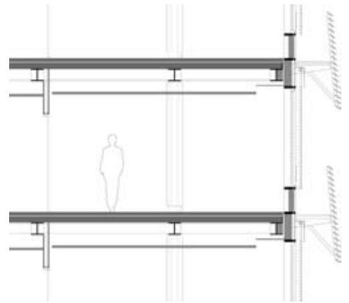
Coupe partielle
